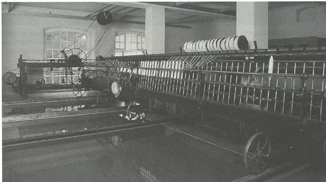
Rheinisches Industriemuseum, Außenstelle Ratingen, Spinning Mule zum Feinspinnen von Garn, um 1845
